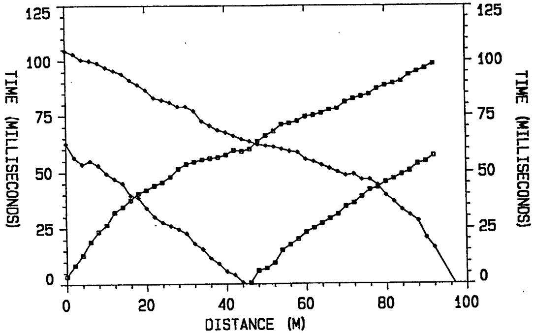
Figure B-2. Refraction data.
